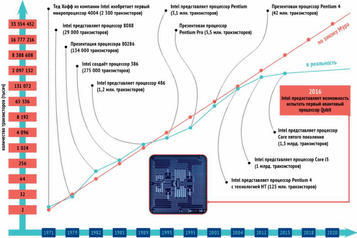
Рис. 6. Зависимость числа транзисторов на микропроцессоре от времени. Видно, что мы переходим от первого закона Мура ко второму. Становятся видны принципиальные ограничения в росте быстродействия компьютеров
