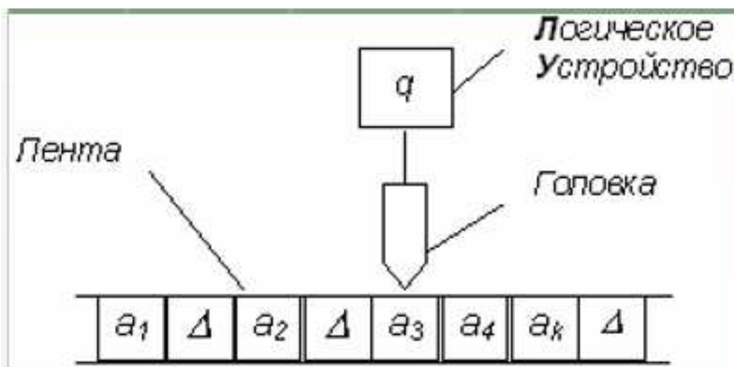
Рис. 3. Машина Тьюринга – основа всей вычислительной техники
