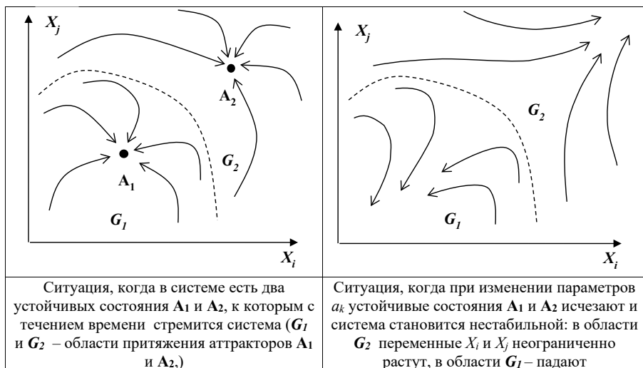
Рисунок 7. Различные виды фазового портрета сложной динамической системы
